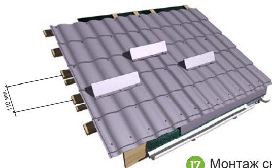
17 Монтаж снігозатримувача
